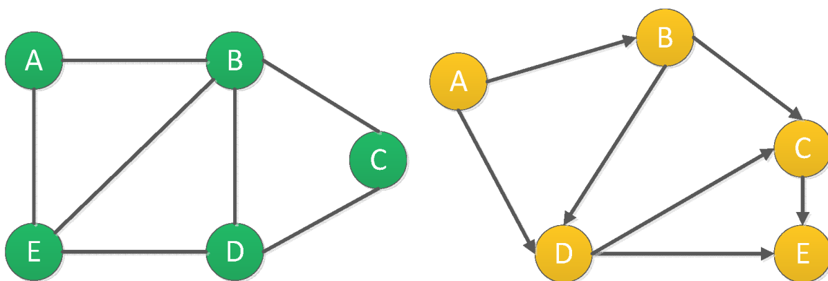
A. 无向图
